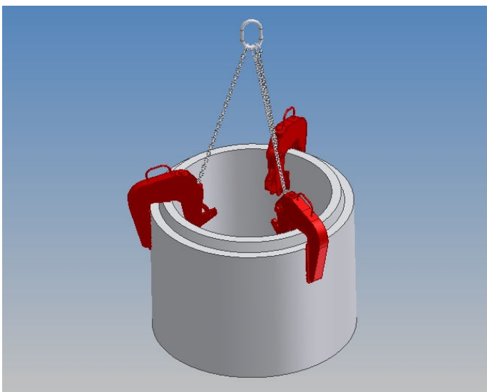
Betongyűrű függeszték
