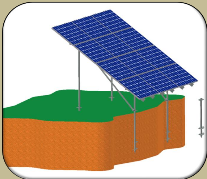
Talajcsavaros alapozás
