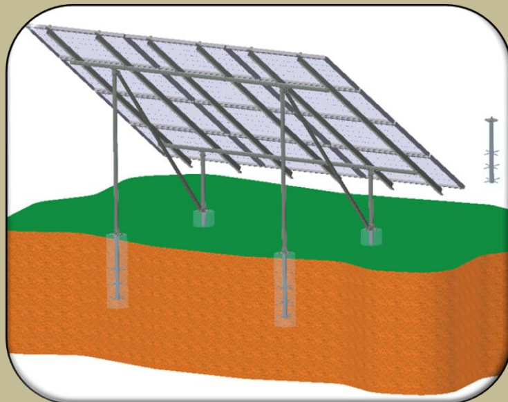
Vasbeton pontalapozás
